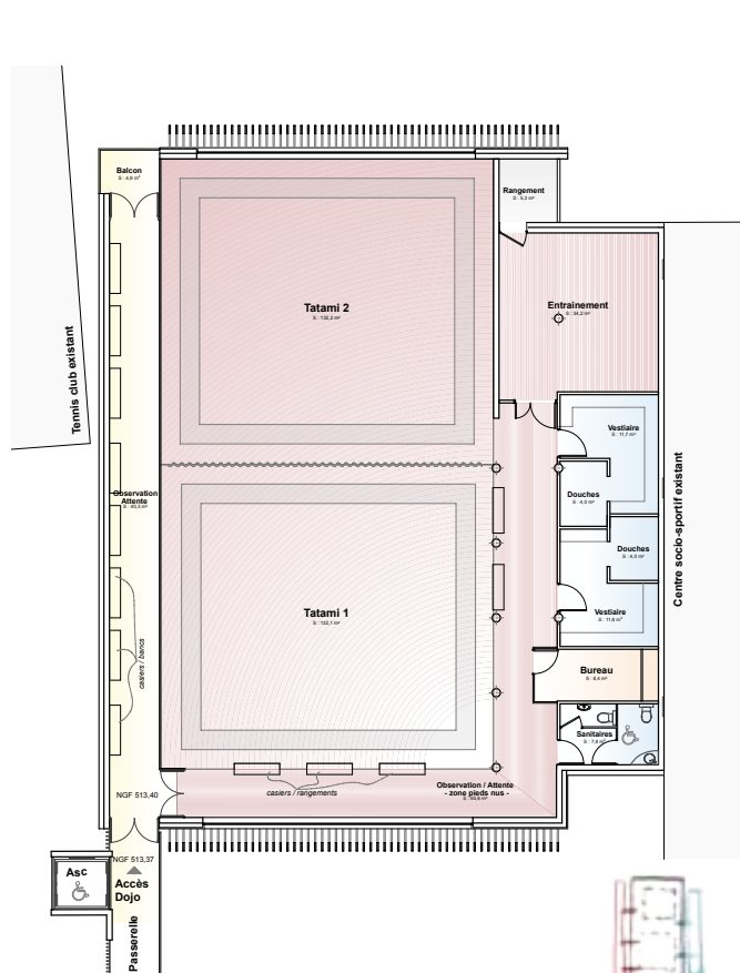
Plan de l'Étage - 1/100e
