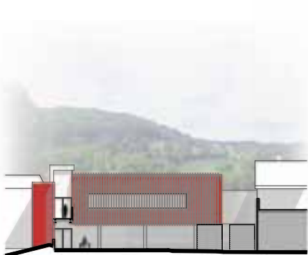
Façade sur la Rue de St Just - 1/200e
